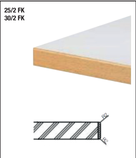
Gerade Standardkante aus Buche 2mm Furnierkante (FK) Echtholz Tischplatte 25 oder 30mm stark Oberfläche HPL Tischplattenkante 2 mm stark, oben und unten gerundet, R 2 mm.
